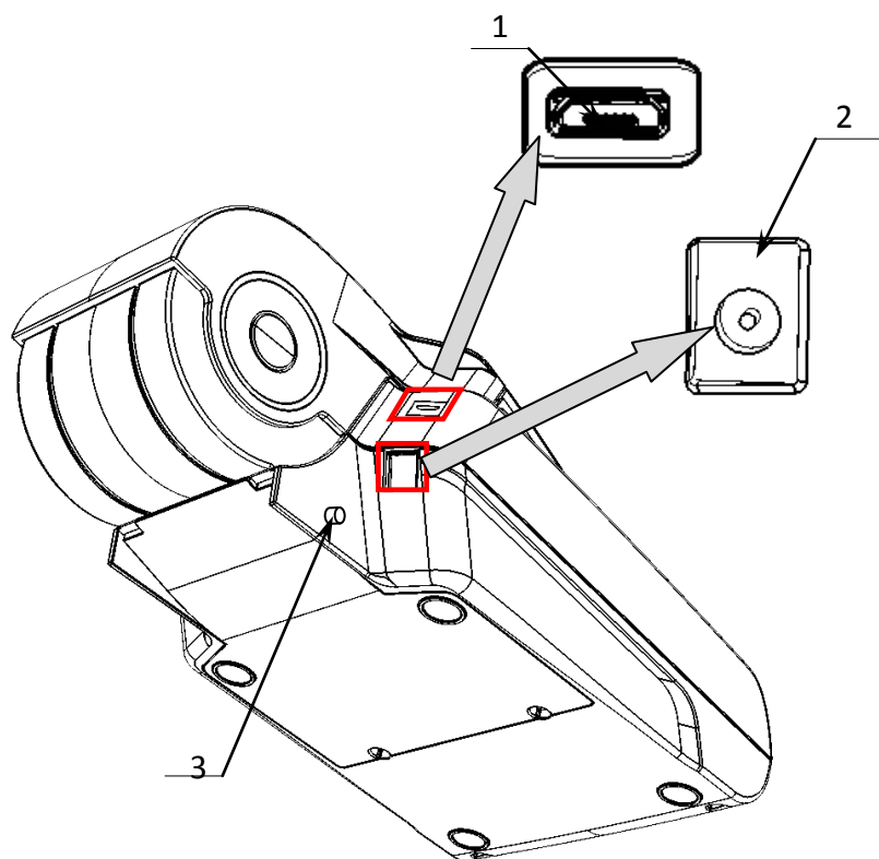
Рисунок 2. Вид сзади/снизу/слева
