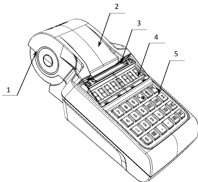
Рисунок 1. Вид спереди/сверху/слева
